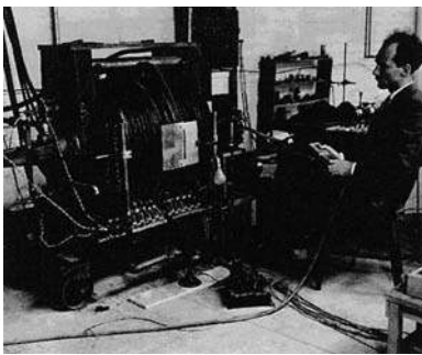
Карл Андерсон в 1931 году в лаборатории Гуггенхайма с конденсационной камерой, в которой ему удалось впервые обнаружить предсказанное Полем Дираком антивещество
