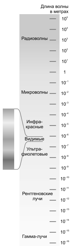
Электромагнитные волны образуют сплошной спектр длин волн и энергий (частот), подразделяемый на условные диапазоны — от радиоволн до гамма-лучей
