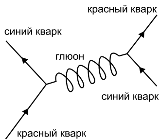
Взаимодействие между кварками в составе элементарных частиц можно графически представить в виде диаграммы Фейнмана, названной так в честь американского физика Ричарда Фейнмана (Richard Feynman, 1918–1988). На представленной диаграмме красный и синий кварки обмениваются глюоном и меняют свой цвет на цвет партнера по взаимодействию
