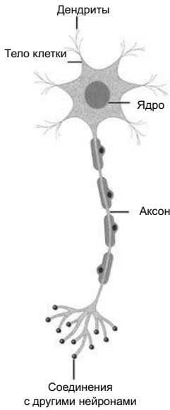
Структура нейрона. Нейроны — важнейшие элементы нервной системы. Эти удлинённые клетки передают нервные импульсы
